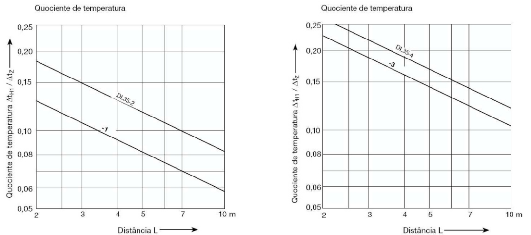
Gráfico 43 □ Quociente de temperatura (Difusor linear 35)
